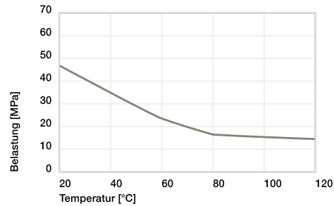
Abb. 02: Maximal empfohlene Flächenpressung in Abhängigkeit von der Temperatur (47 MPa bei +20 °C)
