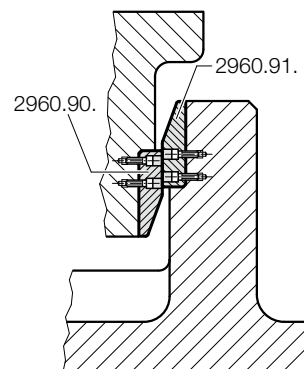
Příklad montáže
