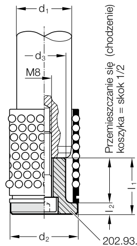
Przykład zabudowy
