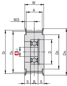
单轴承时
