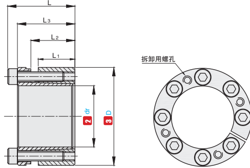
ESTRA 挡圈型（无挡圈安装）
