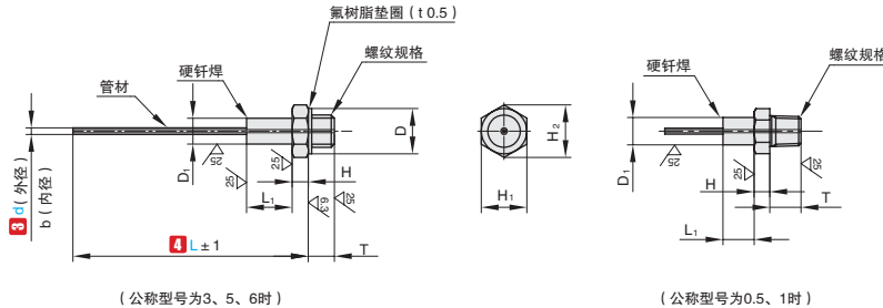
PAWL 外螺纹型
