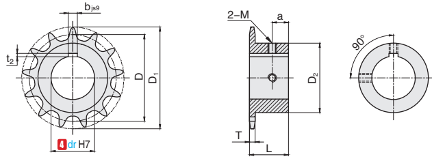
双节距滚子链链轮R型
