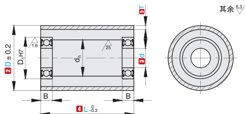
XEPSSN/XEPAN/XEPSSS/XEPAS/XEPSSF/XEPAF 轴承·聚氨酯厚度选择型
