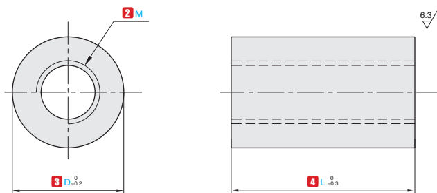
RCMA 内螺纹型
