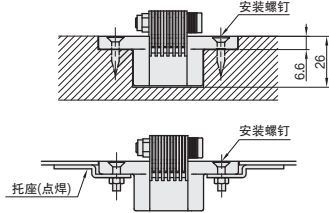
安装图
