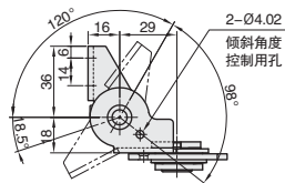
安装加工图
